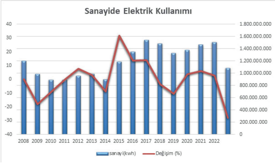
Grafik 3: Sanayide Elektrik Kullanımı
